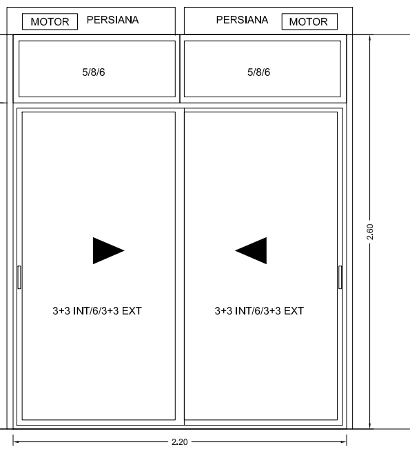
DOS PERSIANAS CON GUÍA CENTRAL
